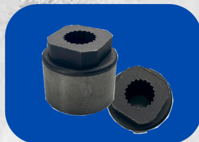
3696 ENGASTADA CATRACA COMP. LM06 LM08 LTR10 LTR12 LF11 62602411
