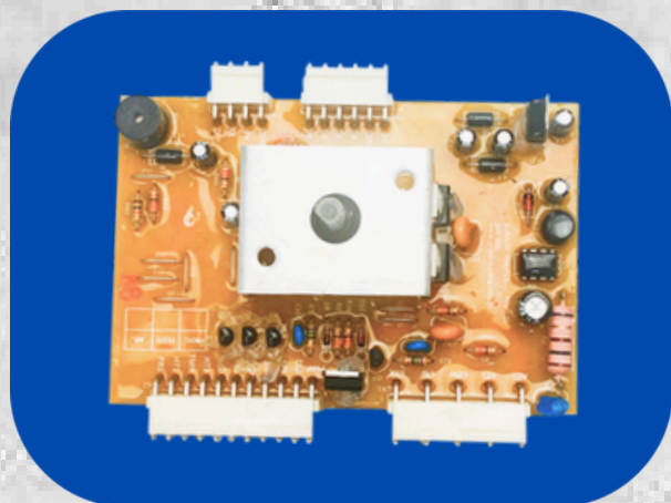
4916 POTÊNCIA COMPATÍVEL LTE12 V3 (70202698)
